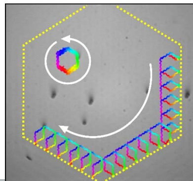
An den Grenzen des Materials bewegen sich die Kunststoffteilchen in ausgedehnten schleifenförmigen Bahnen; im Inneren bewegen sie sich nur in geschlossenen Bahnen und verändern ihre Position kaum. Grafik: Lehrstuhl für Experimentalphysik V, Universität Bayreuth.
